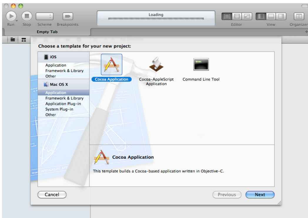
Figure 12.15 : Xcode IDE
