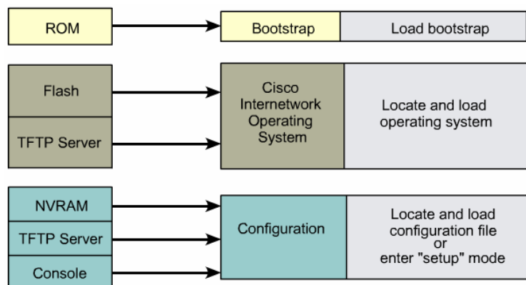
Gambar 2.1 Langkah-langkah inisialisasi di router
