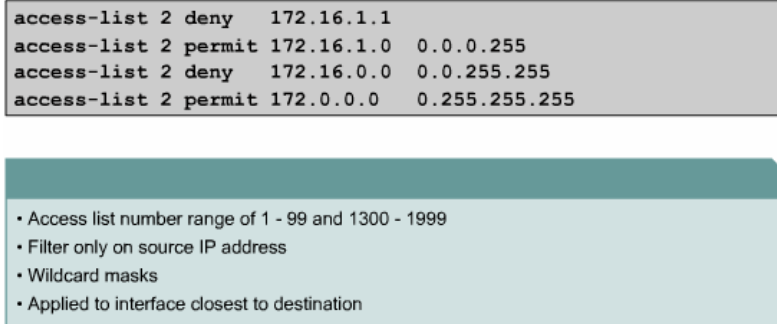
Gambar 2.1 Pernyataan standar ACL
