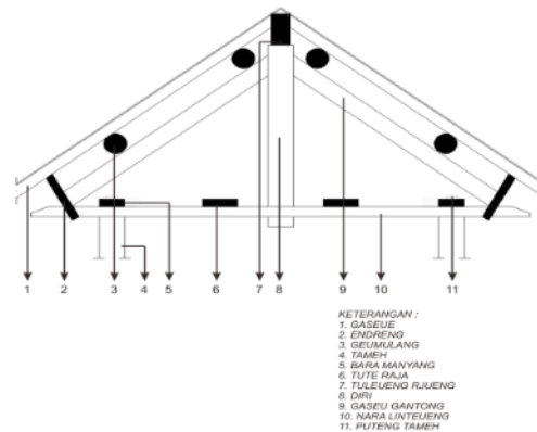
Gambar 12. Konstruksi Rungka
