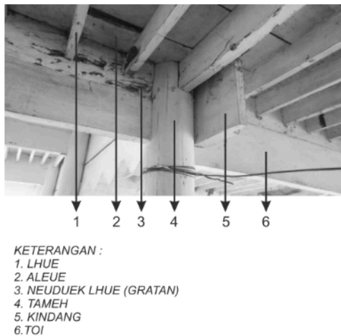
Gambar 13. Sambungan Tiang
