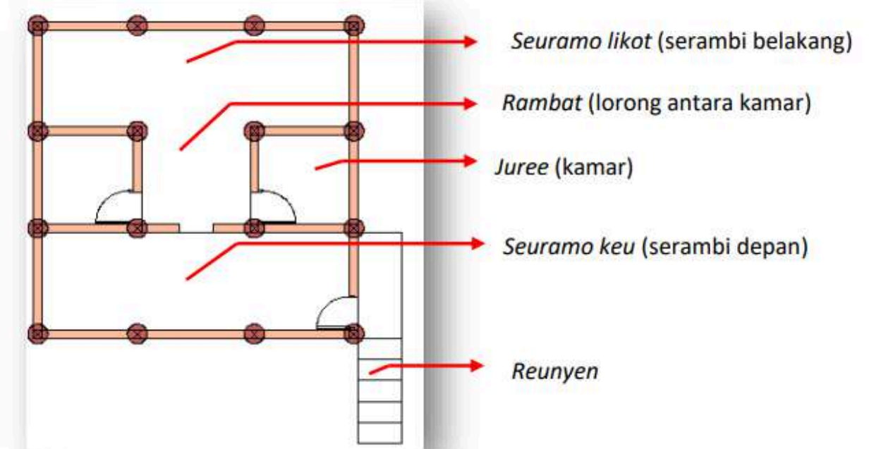
Gambar 6.1. Denah rumoh aceh tipe 1.
