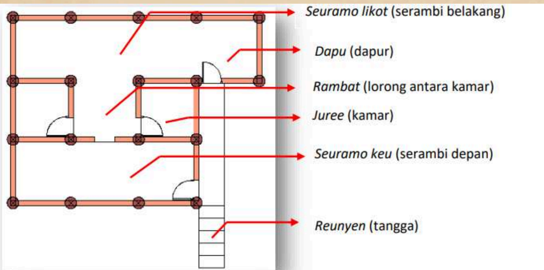
Gambar 6.3. Denah rumoh aceh tipe 2.
