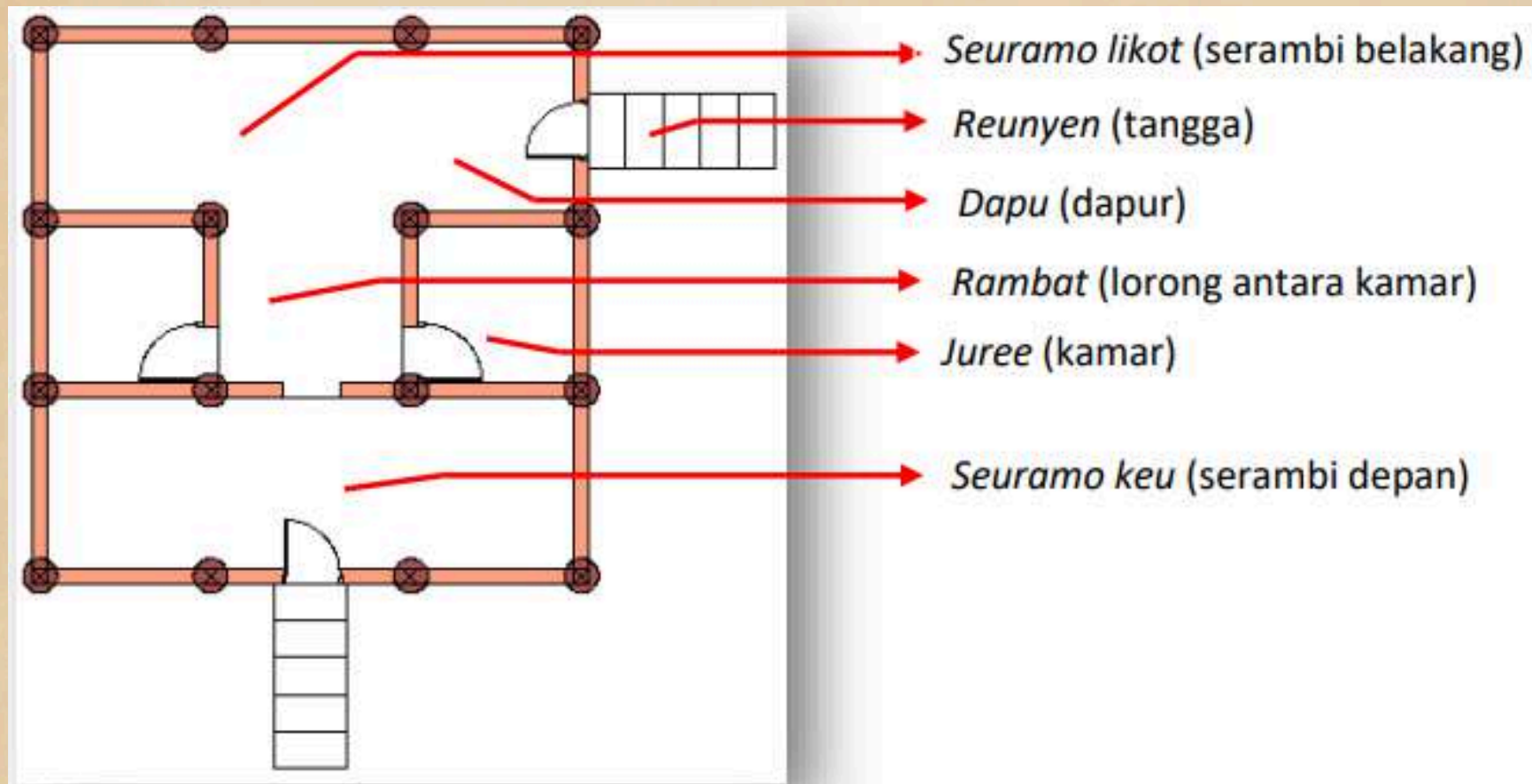
Gambar 6.5. Denah rumoh aceh tipe 3.
